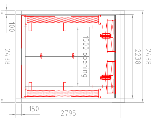
END ELEVATION
