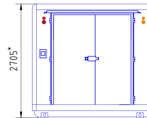
DOOR ELEVATION
